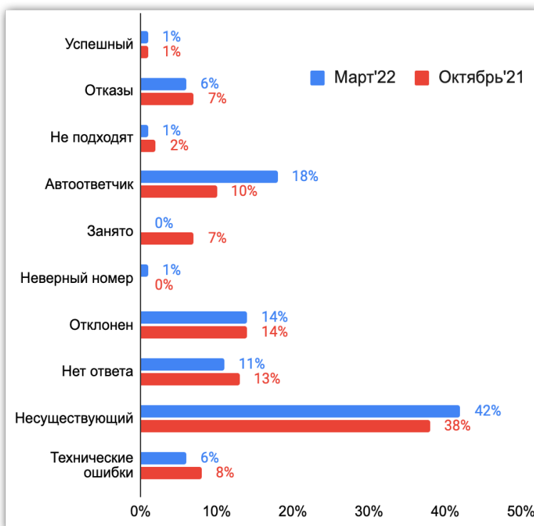
Рис. 1. Динамика статусов попыток контакта с респондентами в ходе общенациональных опросов в РФ (2021–2022)
