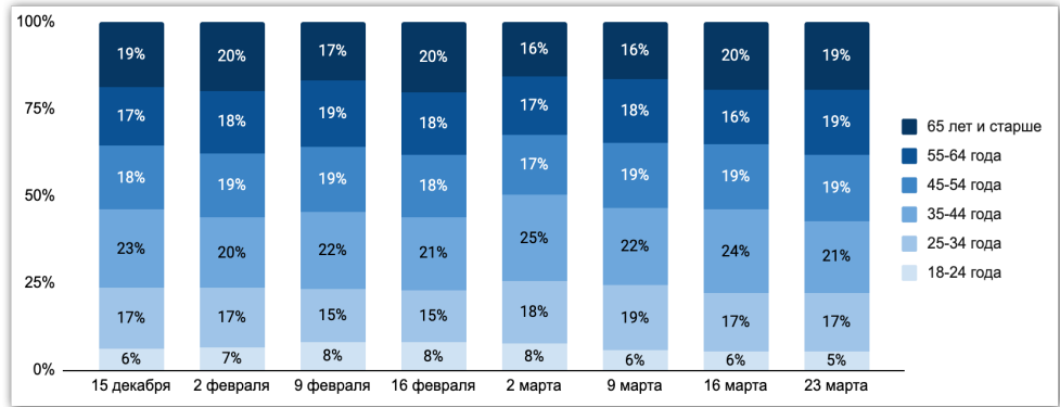
Рис. 2. Динамика представленности в финальной выборке различных возрастных групп в ходе ежедневных опросов «Спутник» (ВЦИОМ, N = 1600, 2021–2022, невзвешенные данные)
