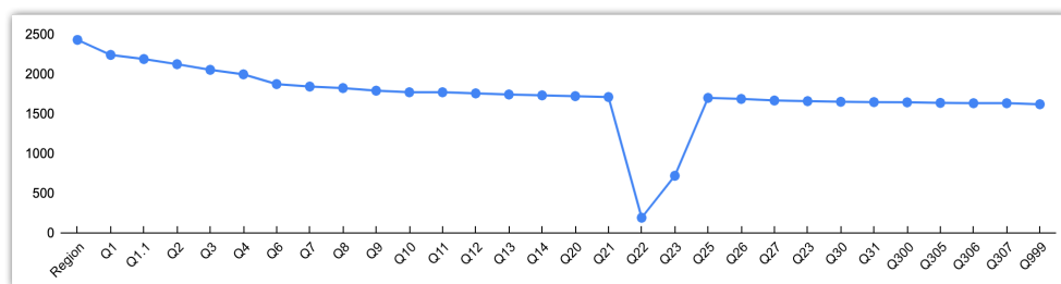
Рис. 4. «Осыпание» объема выборки в ходе телефонного интервью от первого вопроса до последнего ExtremeScan (Опыты, март 2022 г. Вопросы Q22–Q23 задавались только части выборки респондентов)
